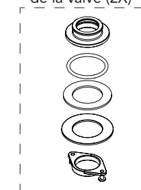
Ensemble du matériel de la valve (2X)
